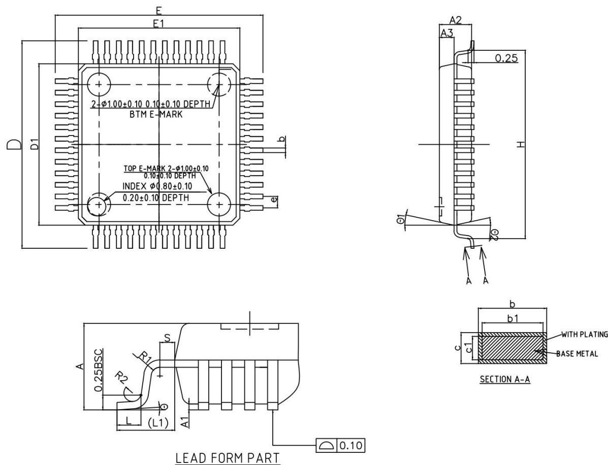
● LQFP48 塑封规格图
